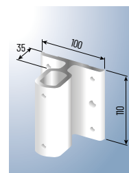
Embase Alu pose en nez de dalle L 100 x H 110 pour Chablis et Irancy
