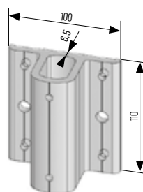
Embase Alu pose en nez de dalle L 100 x H 110 pour Givry et Montagny
